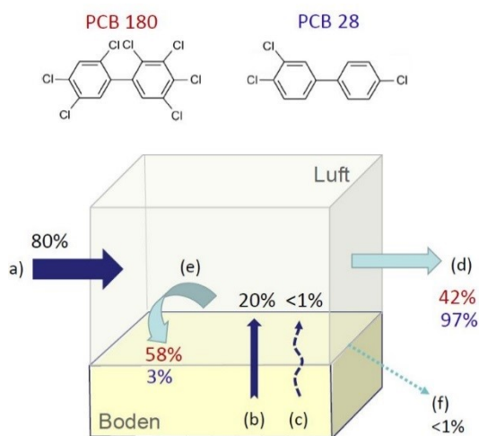
Abbildung 3: Massenbilanz zweier PCB-Kongeneren für die Schweiz. a) Stofffluss aus dem Ausland in die Schweiz, b) primäre Emissionen aus der Schweiz (von Bauprodukten), c) sekundäre Emissionen aus der Schweiz (Remobilisierung von deponierten Molekülen), d) Stofffluss von der Schweiz ins Ausland, e) Deposition auf Böden. Grafik adaptiert (Glüge, Bogdal, Scheringer, & Hungerbühler, 2016).
