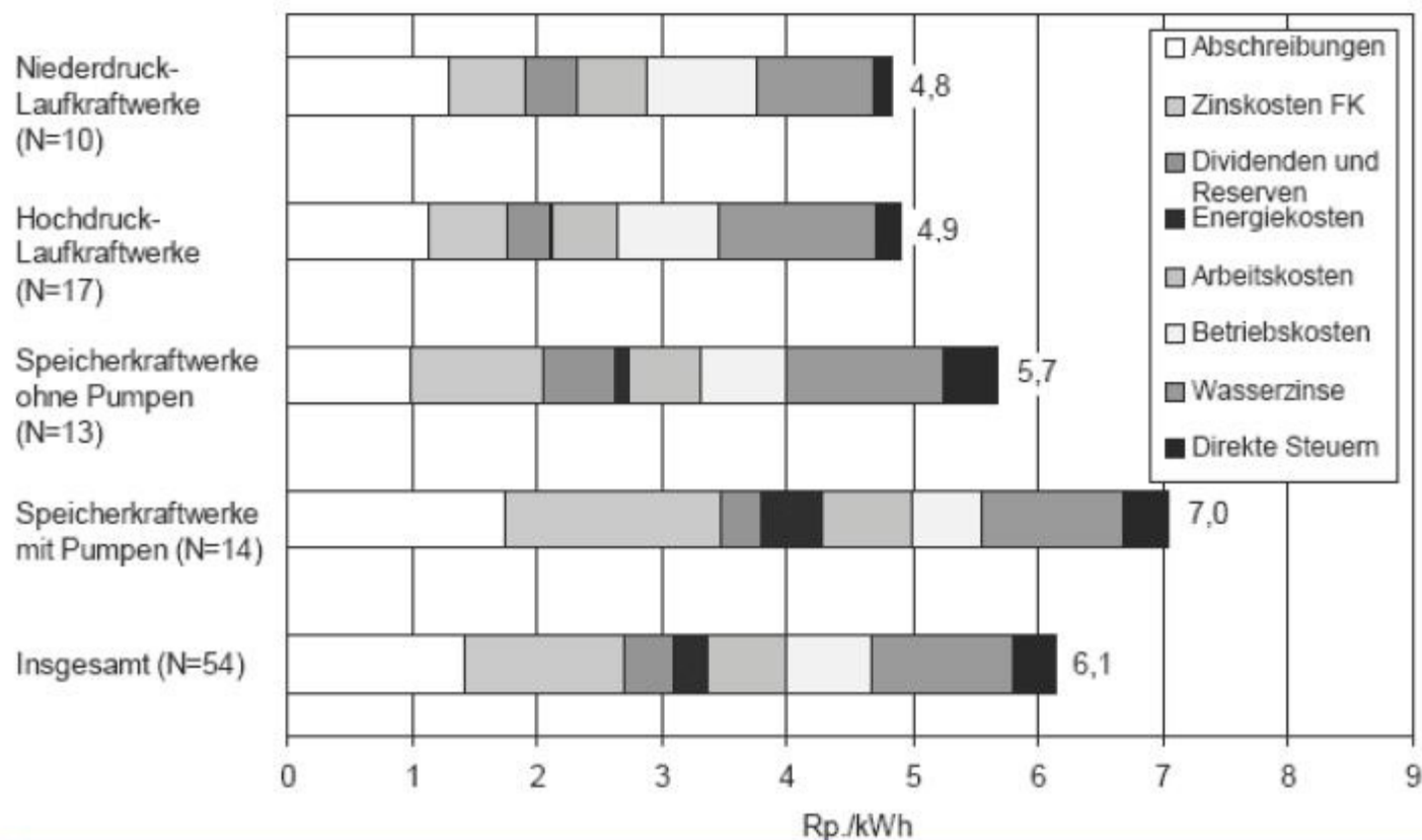
Figur 5: Die Gestehungskosten pro Kraftwerktyp und kWh Strom (Quelle: Banfi et al. 2004).
